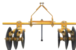
Barra Portaherramienta Permite el desplazamiento de la torre y las secciones.
